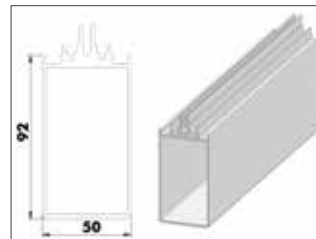
Sparren 100 mm
