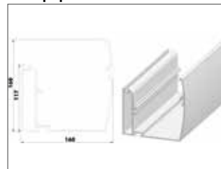
Rinne 160 mm
