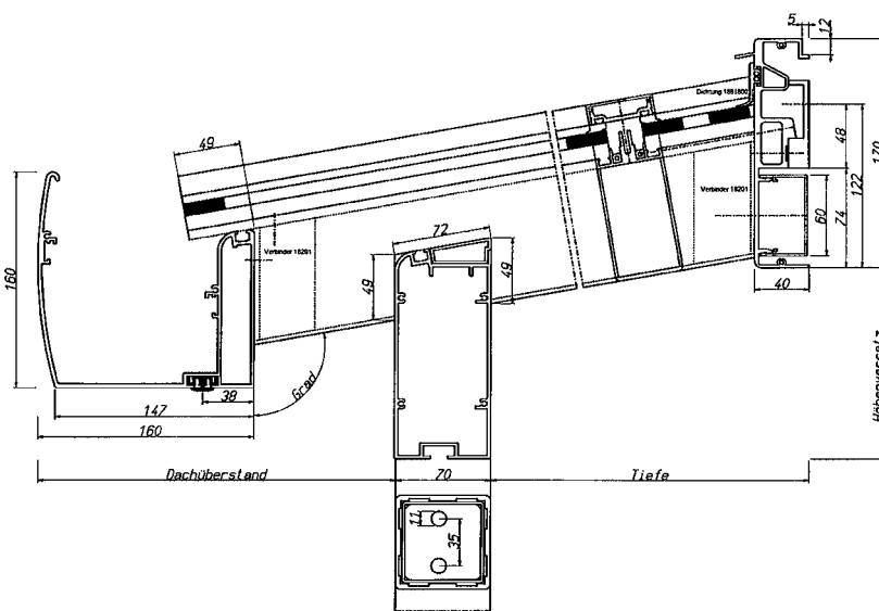
Rinne 160 mm
