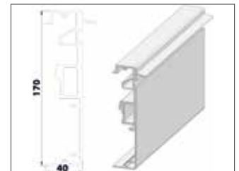
Wandanschluss 170 mm
